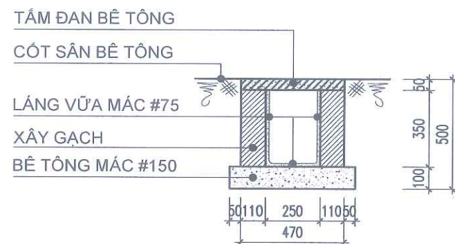
CHI TIẾT RÃNH THOÁT NƯỚC HIỆN TRẠNG L = 170M
