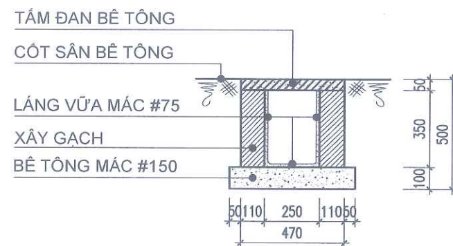
CHI TIẾT RÃNH THOÁT NƯỚC XÂY THÊM
