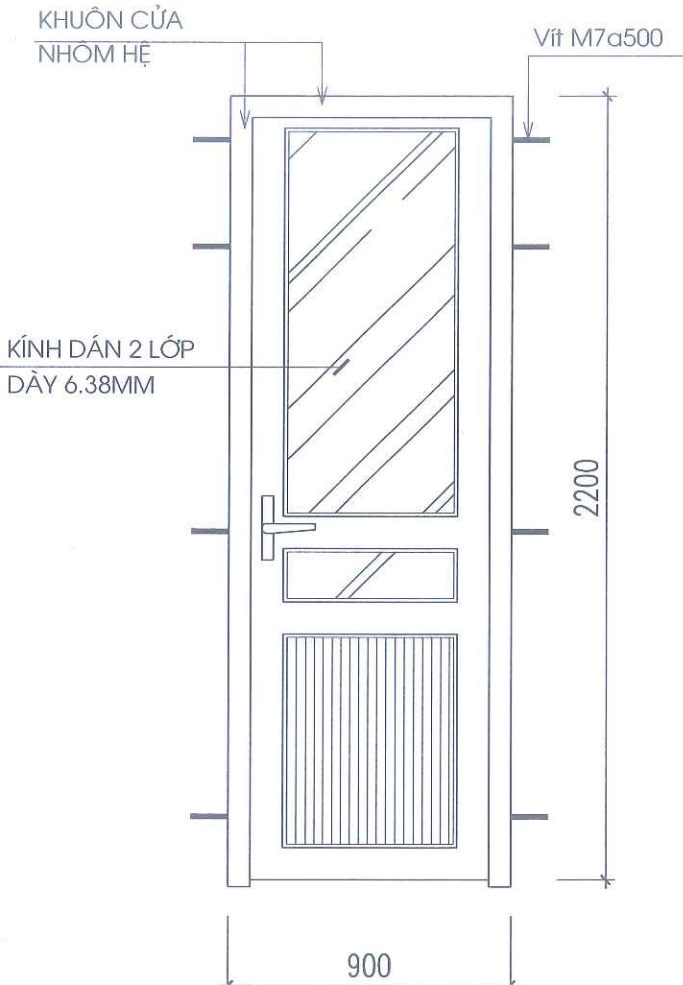
CỬA Đ2M (THAY THẾ DC) (SL: 1 CK )
