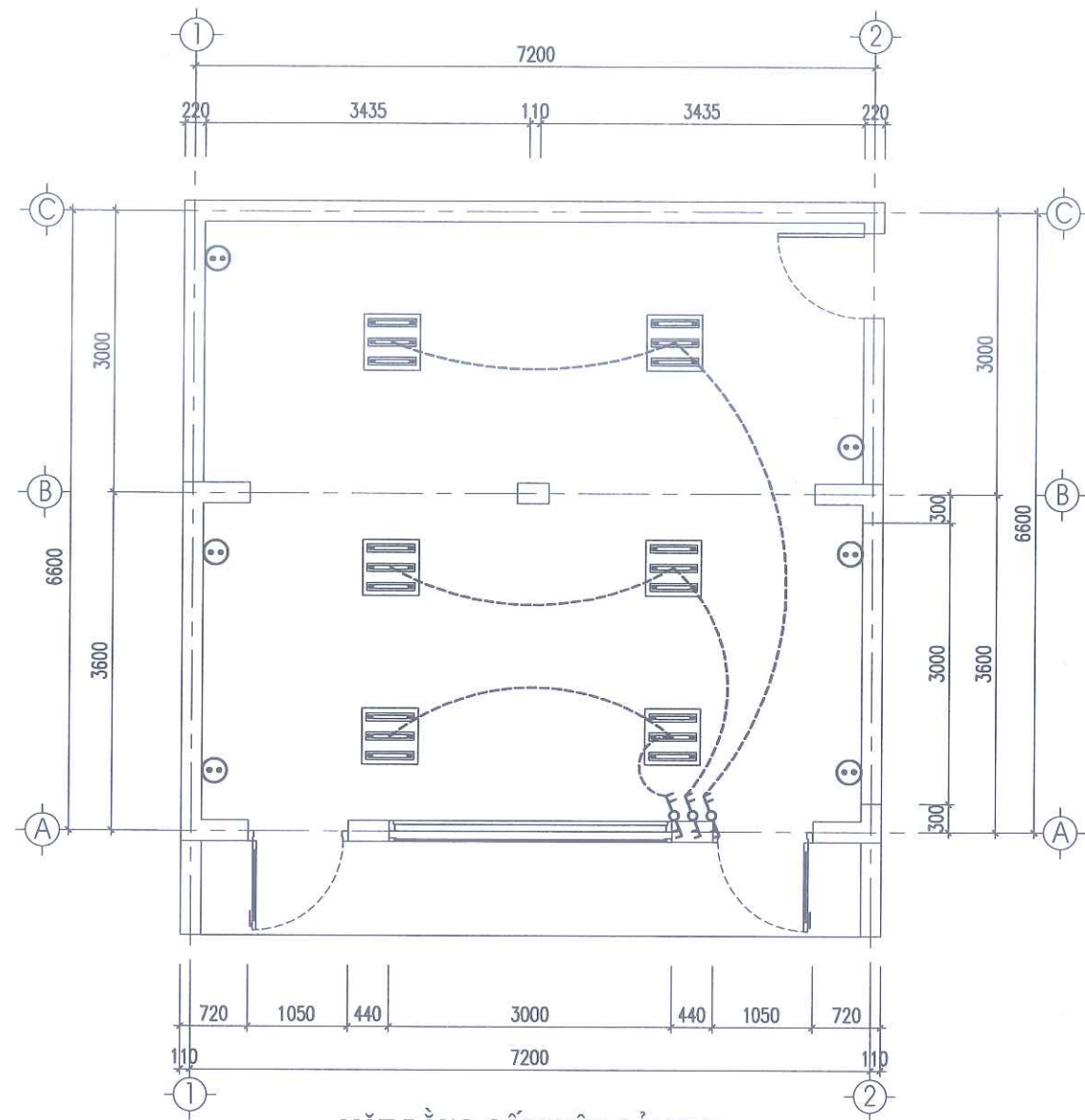
MẶT BẰNG CẤP ĐIỆN CẢI TẠO
