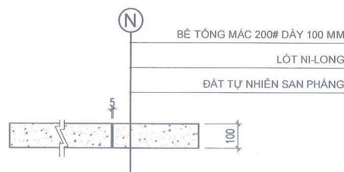
MẶT CẮT CHI TIẾT SÂN DÀY 100MM
