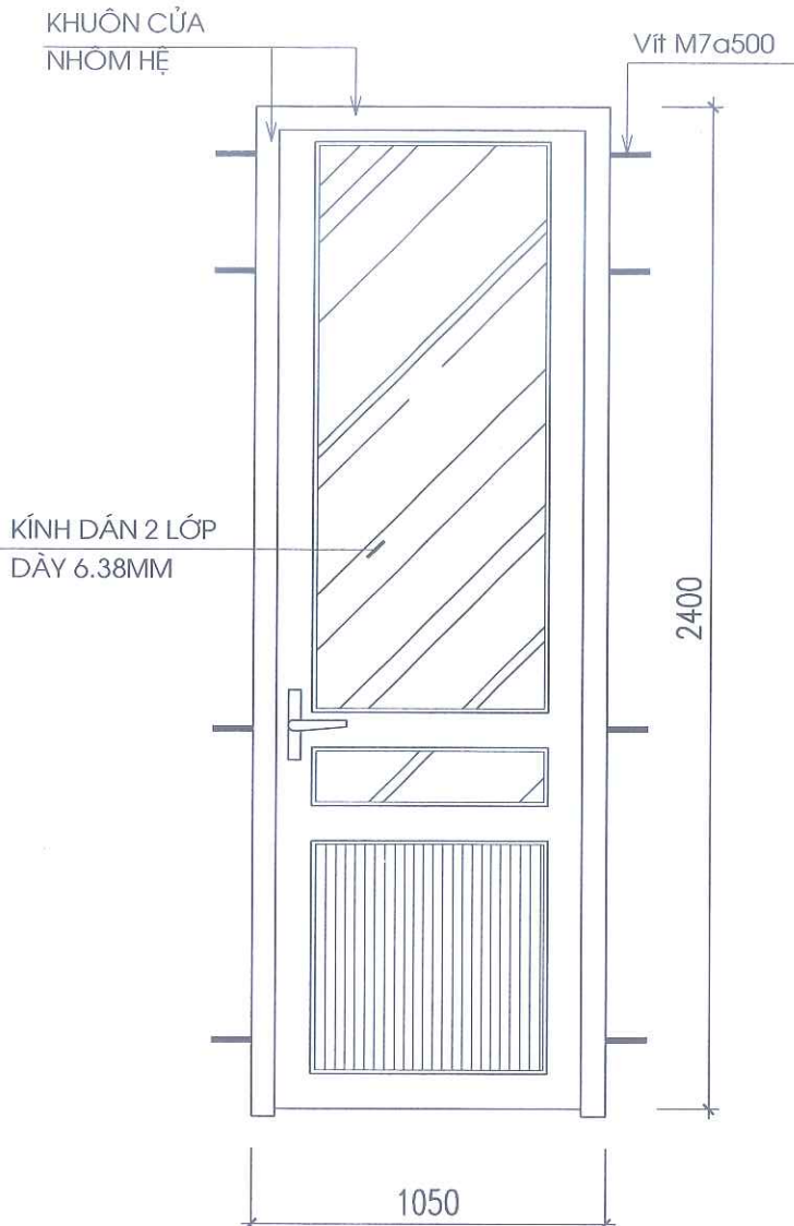
CỬA Đ1M (THAY THẾ VKK1) (SL: 2 CK )
