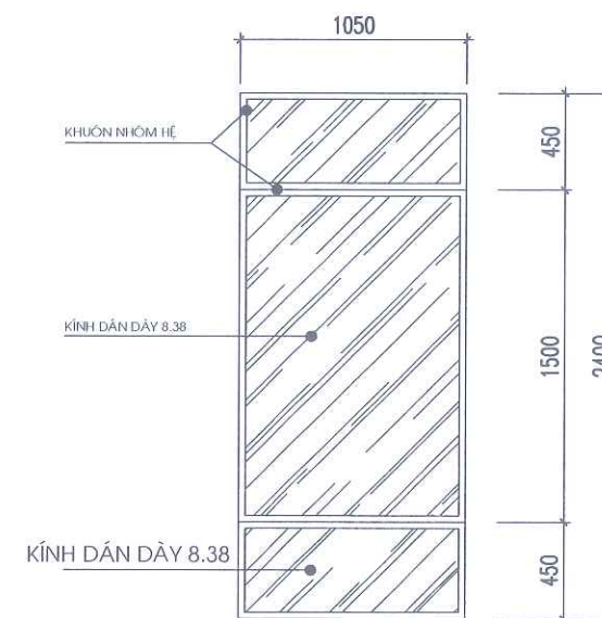
CHI TIẾT VÁCH KÍNH VK1 (02 CK)
