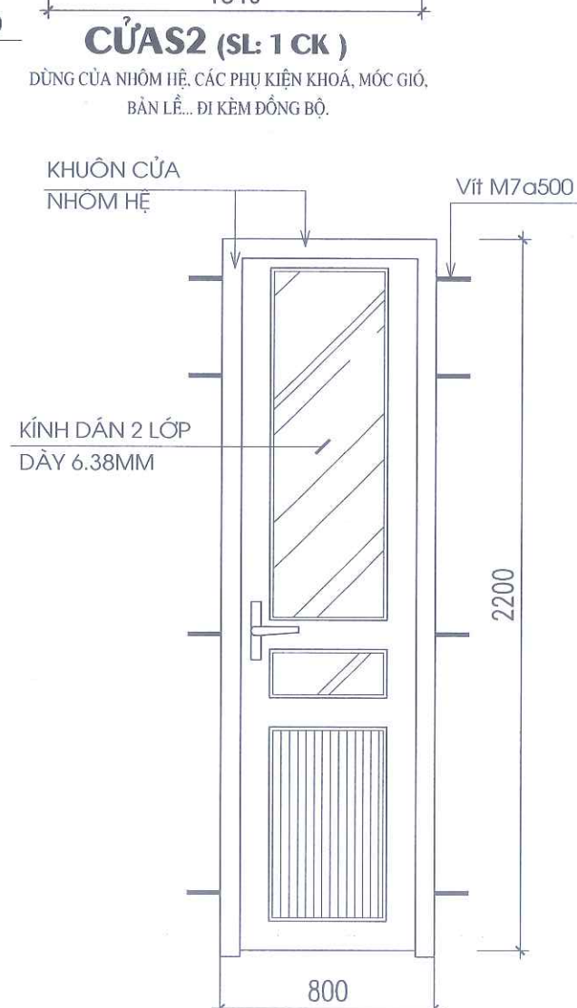
CỬA Đ2 (SL: 04 CK )
