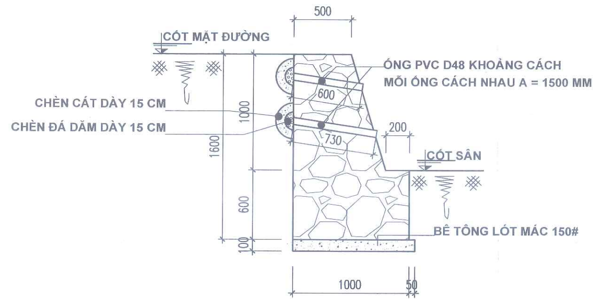
MẶT CẮT KÈ CHẶN ĐẤT
