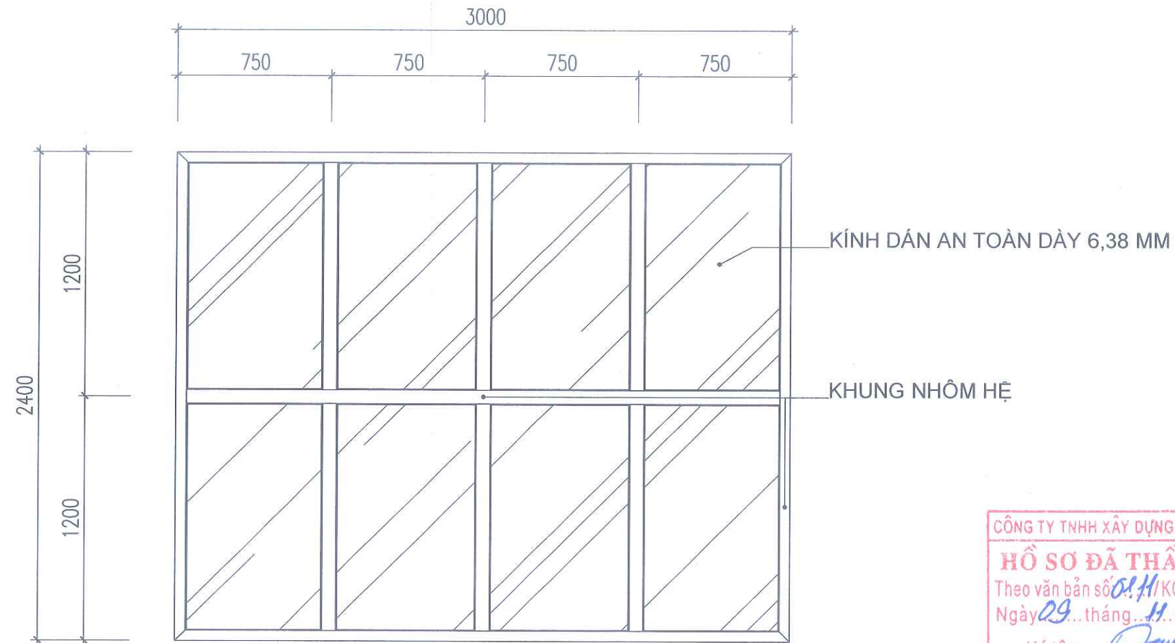
VÁCH KÍNH VKM THAY MỚI (SL: 01 C.K)
