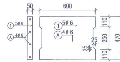
TẦM ĐAN BÊ TÔNG (SL: 38 TẦM)
