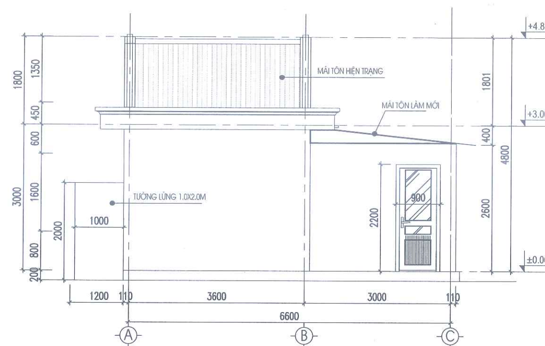
MẶT ĐÚNG CẢI TẠO TRỰC A - B
