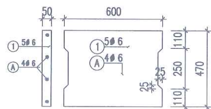
TẦM ĐẠN BÊ TÔNG (SL: 170 TẦM)
