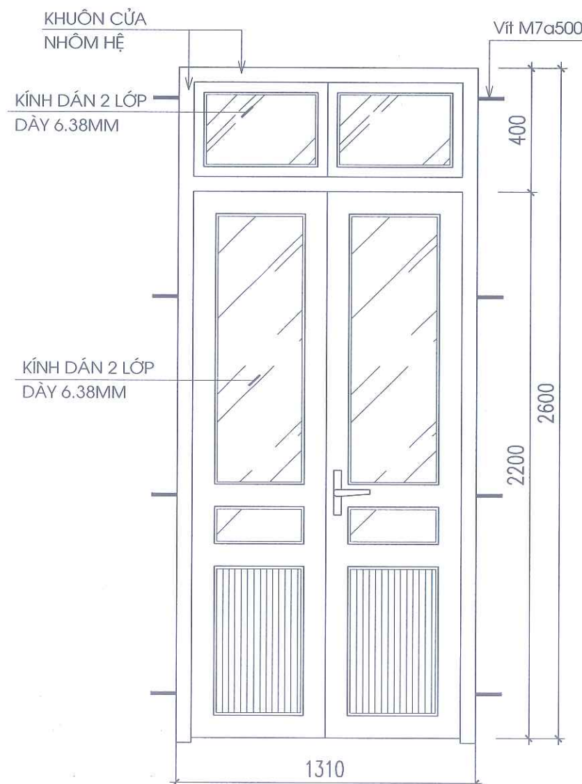
CỬA Đ1 (SL: 14 CK )
