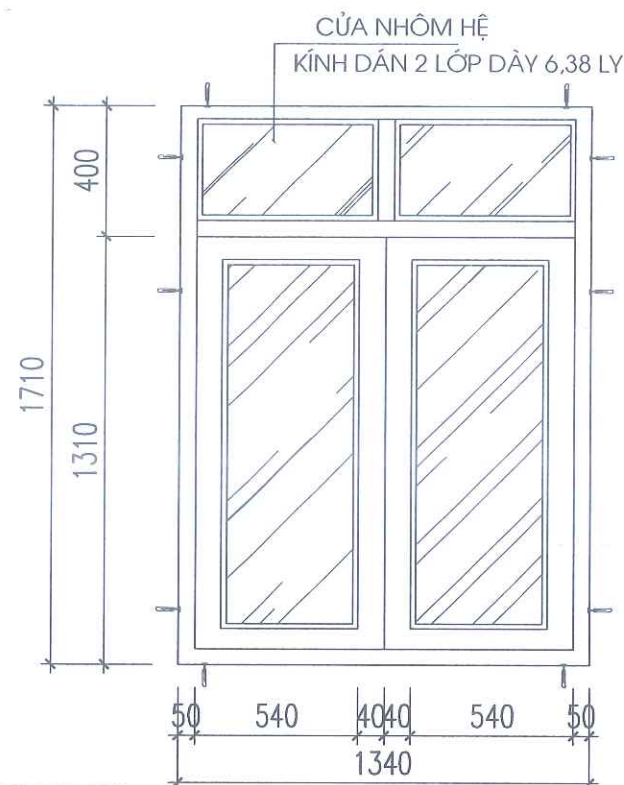
CỬA S2 (SL: 1 CK )
