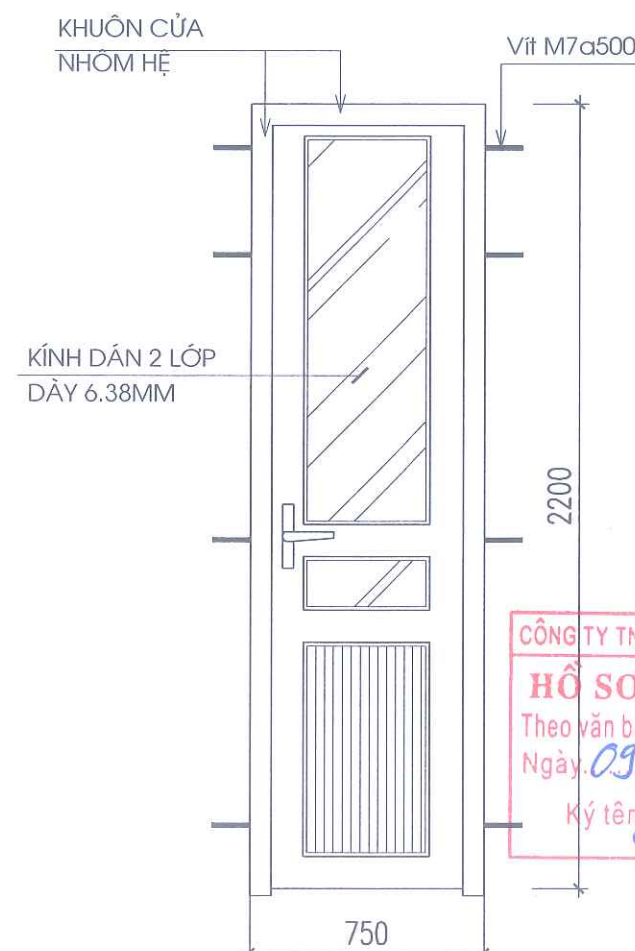
CỬA Đ3 (SL: 04 CK )
