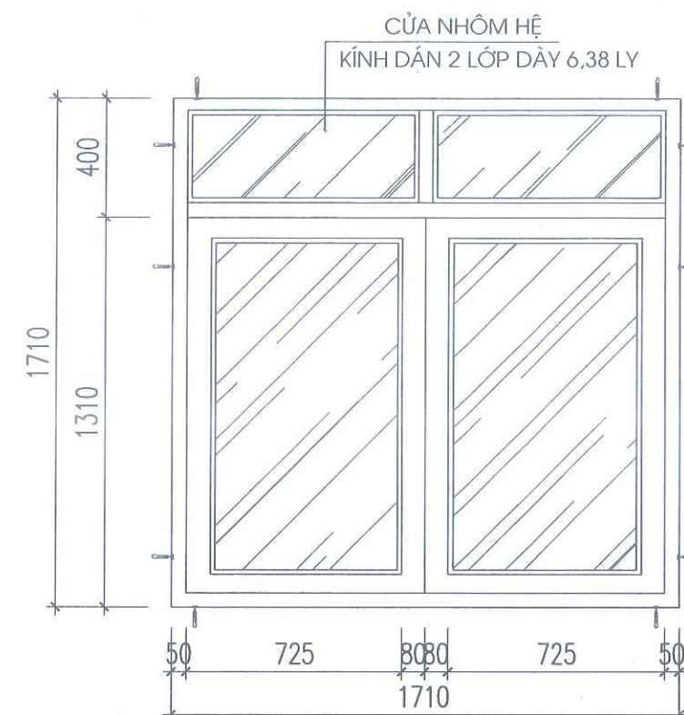
CỬA S1 (SL: 16 CK )
