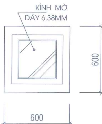
CỬA S3 (SL: 04 CK )
